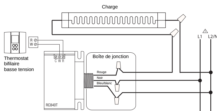
Figure 1 : Connexion typique du relais et d'un thermostat bifilaire de basse tension
