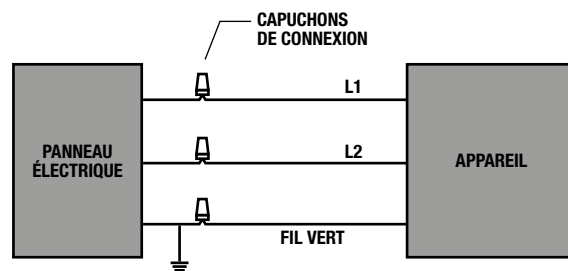
DIAGRAMME ÉLECTRIQUE DES COMPOSANTES
